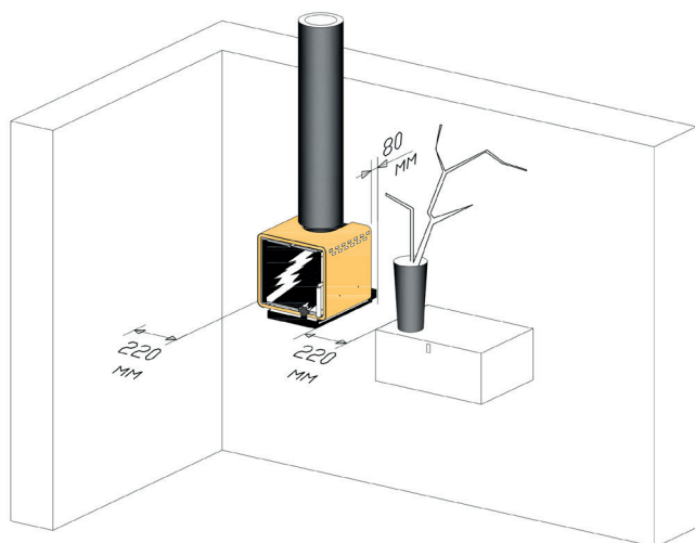
Пожаробезопасные отступы*
