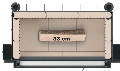
Топка с меньшей глубиной установки
