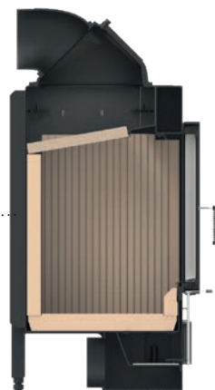
Глубокая топка НАКА 37/50G
