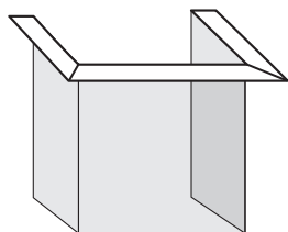
Монтажная рама с 3 сторонняя Ширина 70 мм Толщина 4 мм Толщина 8 мм (УКА 37/125/37/57)
