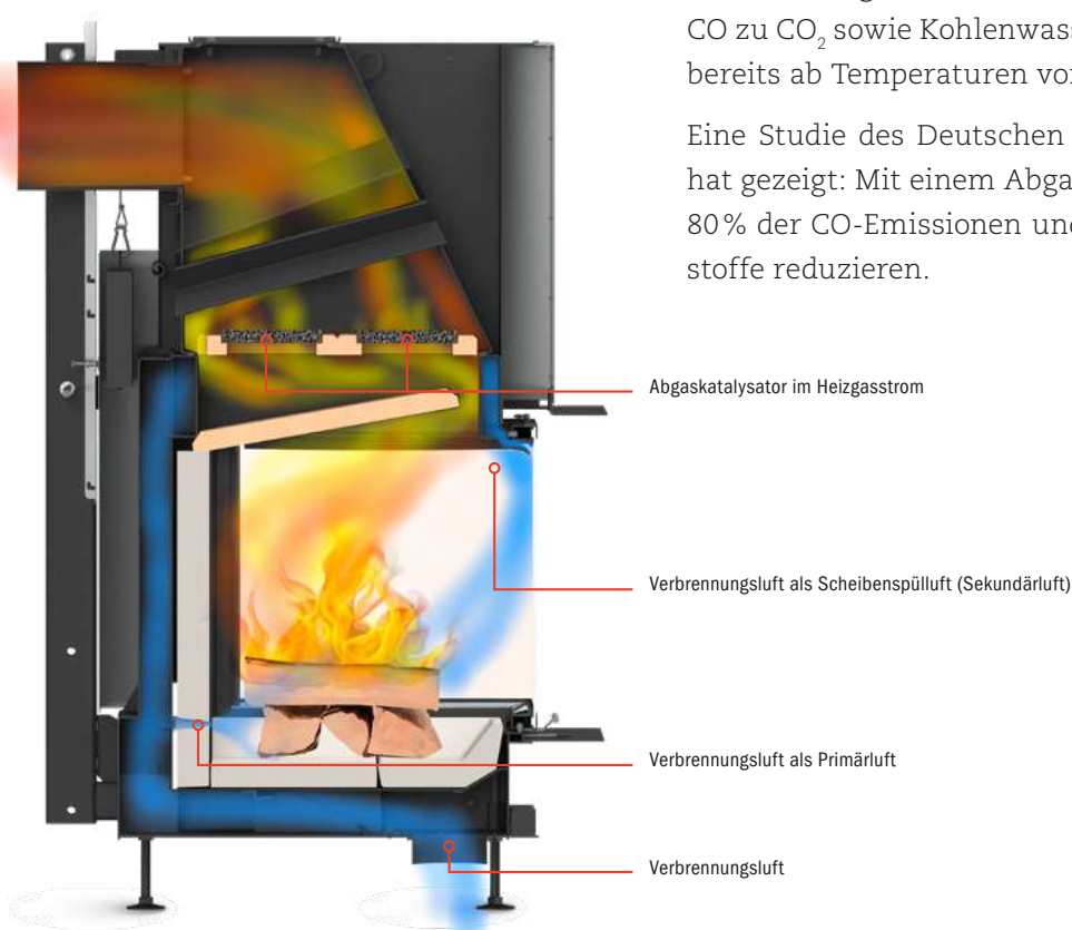
Schnitt durch den Panorama-Kamin 51/50/50/50 mit integriertem Abgaskatalysator
