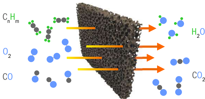
Katalysator im Betrieb ab 250^\circ\text{C}
